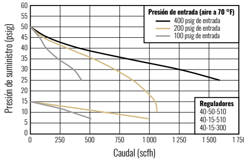
Gráfico de caudales de baja presión para Series 40™
