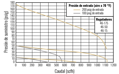
Gráfico de caudales para Series 46™
