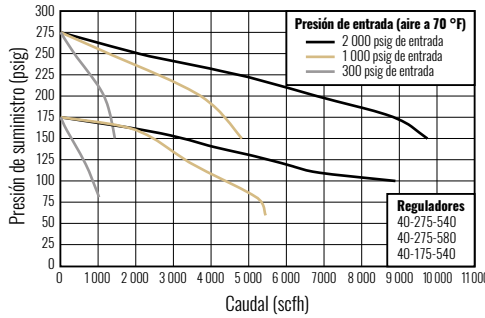
Gráfico de caudales de baja presión para Series 40™
