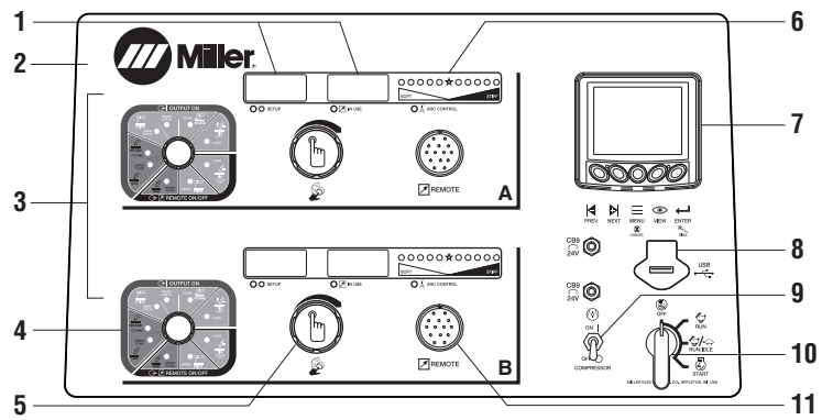
Panel de control (todos los modelos)
