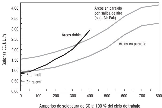
Curva de consumo de combustible
