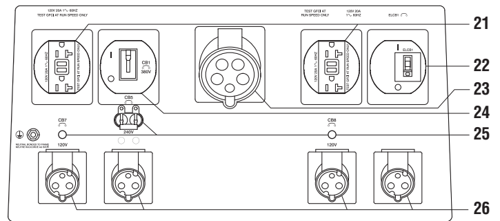
Tomacorrientes y disyuntores (modelos internacionales)
