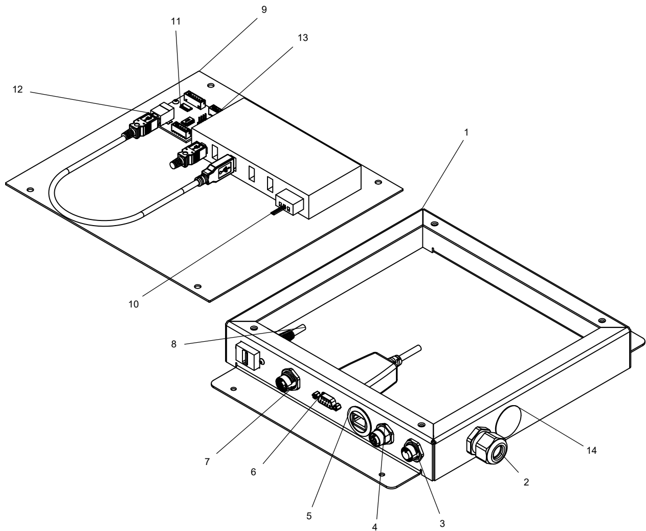
Controller Top Hat Assembly
